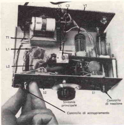
La posizione in cui si trova il telaio ausiliario sul telaio principale è messa in evidenza da questa foto dell'unità completa. I controlli di sintonia principale e di reazione sono accoppiati rispettivamente agli alberi dei condensatori C1 e C2.
