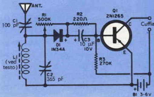
Fig. 3 - Circuito del ricevitore per onde medie. Notate l'uso della polarizzazione diretta sul diodo.
