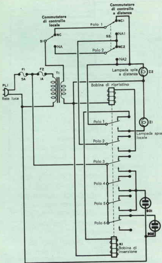
Circuito elettrico del dispositivo che serve a controllare a distanza un sistema fonoriproduttore.
