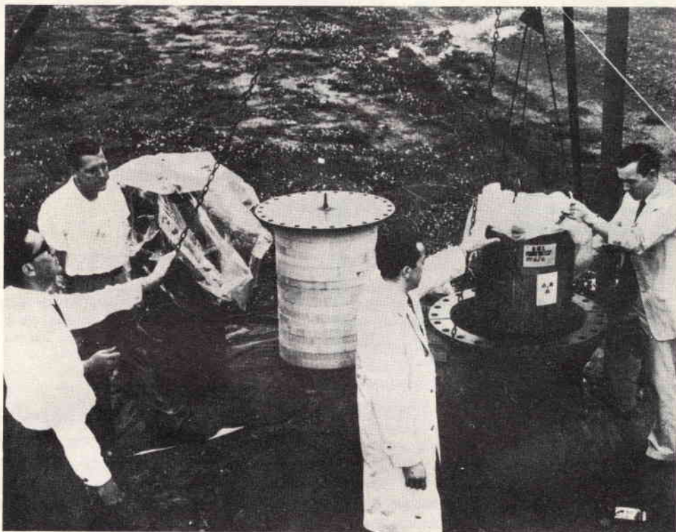
In fotografia si vede il generatore per la stazione, posto in un cilindro semiinterrato, durante le prove effettuate a Baltimora (U.S.A.) presso la fabbrica della Martin Company. Quando la stazione automatica sarà installata funzionerà per due anni senza manutenzione e rifornimento.
