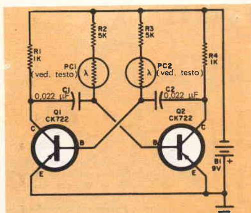
Fig. 4 - Questo multivibratore è sensibile alla luce che controlla la frequenza di funzionamento.
